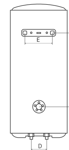
Вид сзади
