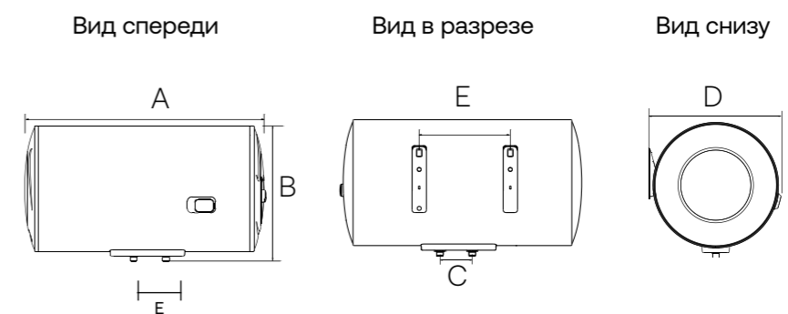
Габаритные размеры (мм)
