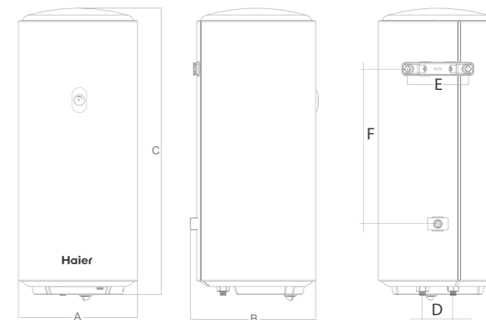
Габаритные размеры (мм)
