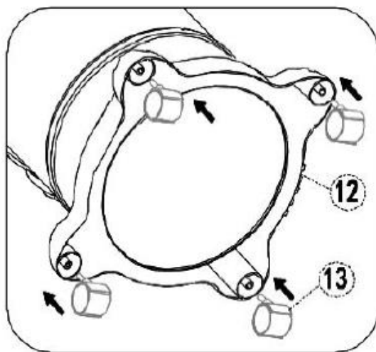
Сборка колес
