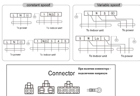
Рис. 21 Подключение наружного блока.
