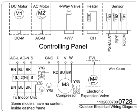
Рис. 24 Электрическая схема для наружных блоков мощностью 7 000, 9 000, 12 000, 18 000, 24 000 BTU, переводы см. таблицы 9-10.
