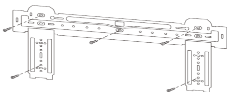
Рис.5 Монтажная пластина
