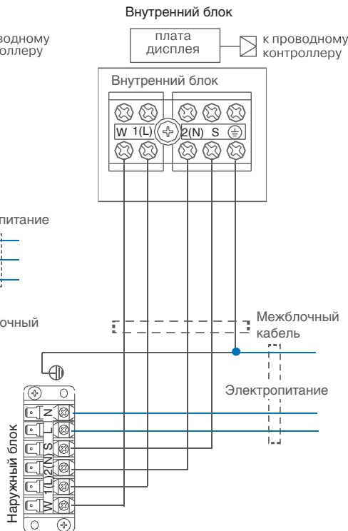
Подключение электропитания к наружному блоку (модели 9-12-18 kBTU) Не рекомендуемая схема!
