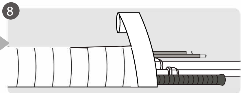
8 Выполните обмотку трассы монтажной лентой
