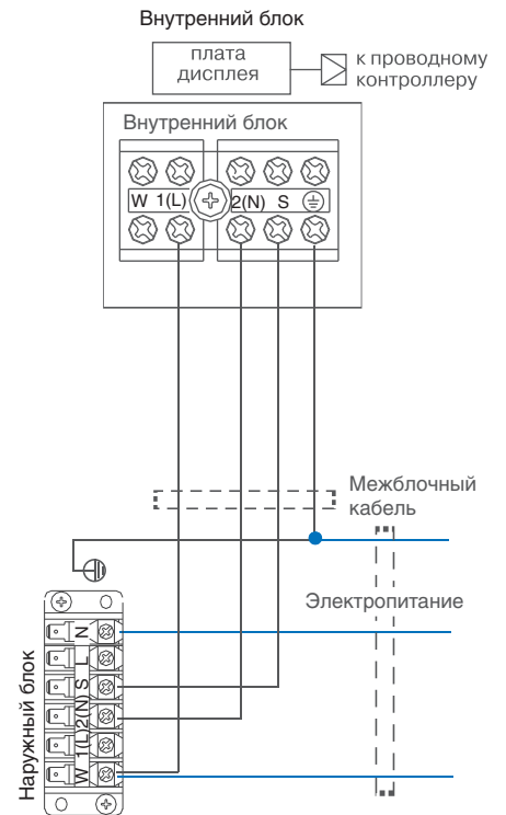
Подключение электропитания к наружному блоку (модель 24 kBTU)
